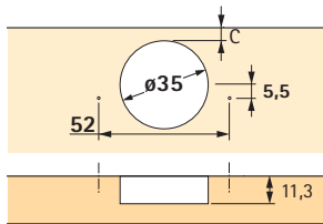
Bohrmaße T42
