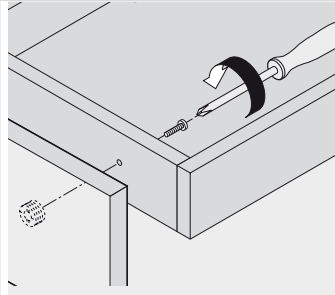
Schroef M4x20 gebruiken
