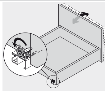
560/566/561: schuine via de glijder
