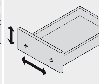
Verstelling hoogte/zijde via frontver- stelbeslag \pm 2 mm
