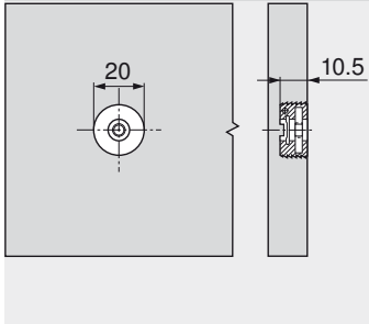
Matrijs voor MINIPRESS + PRO-CENTER MZM.0095
